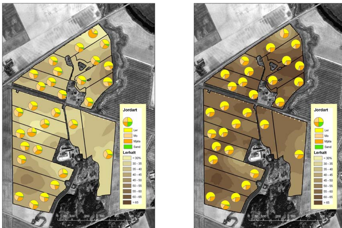
Figur 2. Jordart (lera, mjåla, mo och sand, %) i provtagningspunkterna i matjord (till vänster) och alv (till hger) vid karakteriseringen med interpolerad lerhalt (%) och K-HCl ( \text{mg g}^{-1} ) i bakgrunden.
