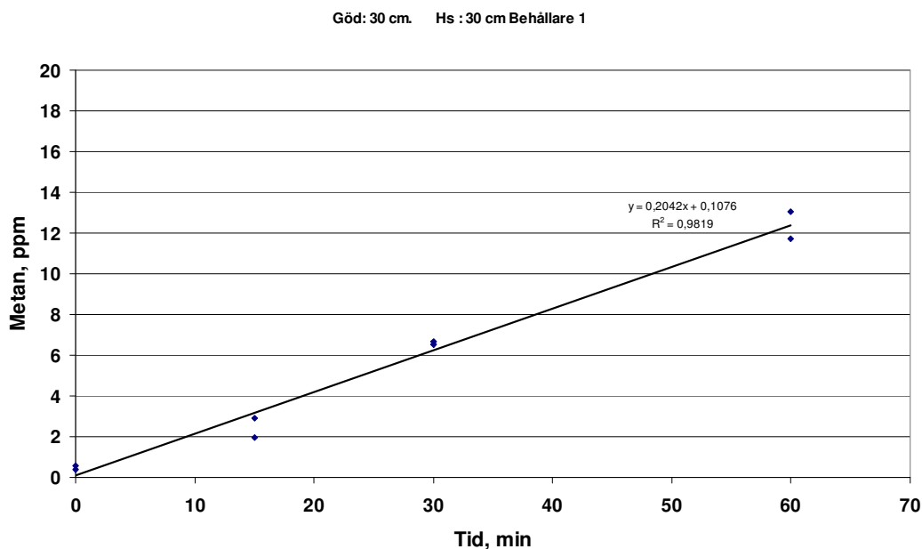
Bild 4. Gaskoncentrationer av metan hos uttagna prov vid olika tider efter förslutning. Behållaren var fylld med 30 cm gödsel och det var 0,3 m i höjd mellan gödselyta och lock.
